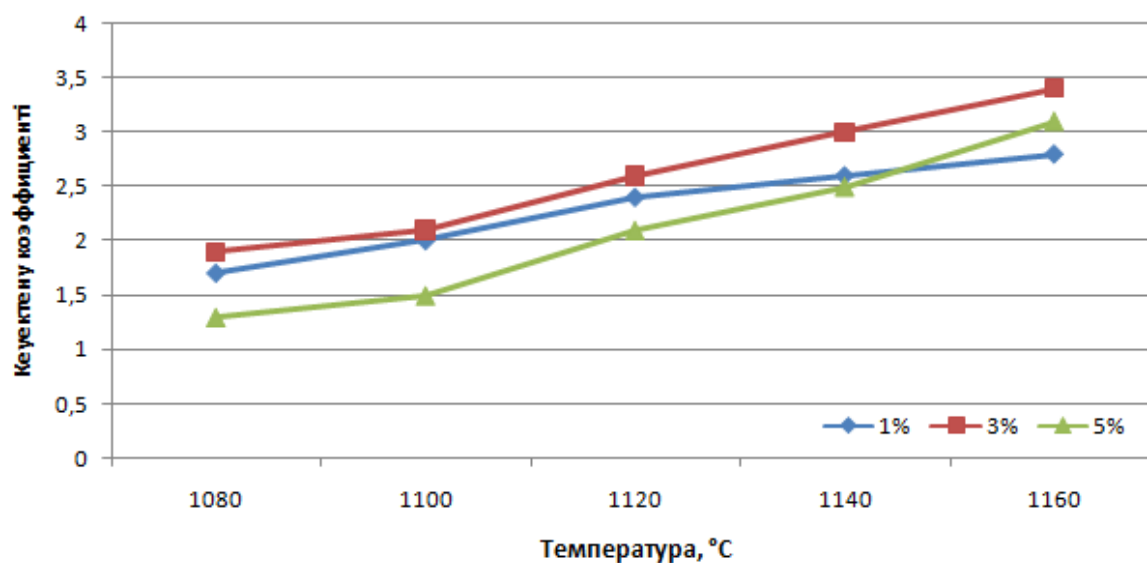
Сурет 1 - Күйдіру температурасына тәуелді Қыңғырақ-Келес бентонит сазы мен ағаш үгіндісі негізіндегі керамогрануляттардың кеуектену коэффициентінің өзгеруі
