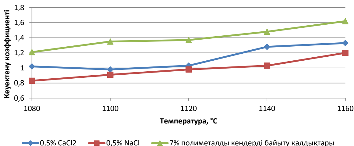
Сурет 1 - Күйдіру температурасына тәуелді Қыңғырақ-Келес бентонит сазы мен минералды қоспалар негізінде алынған керамогрануляттардың кеуектену коэффициентінің өзгеруі
