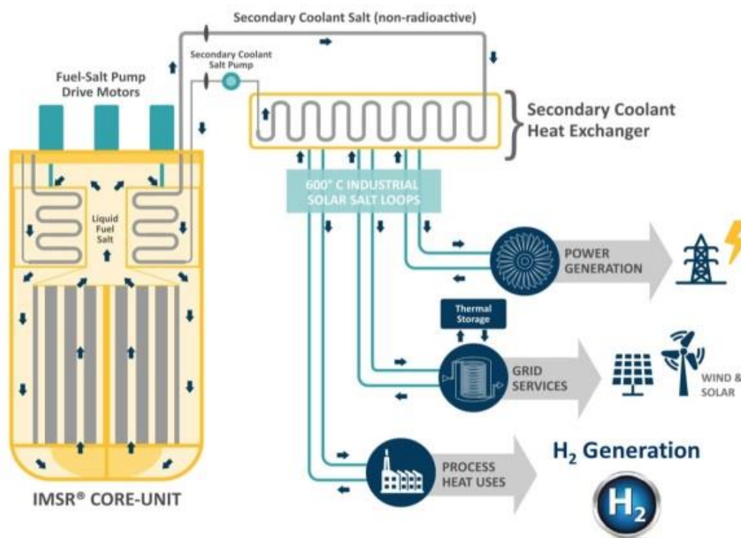
Рис.1. Производство водорода с интегрированным реактором на расплавленных солях IMSR
