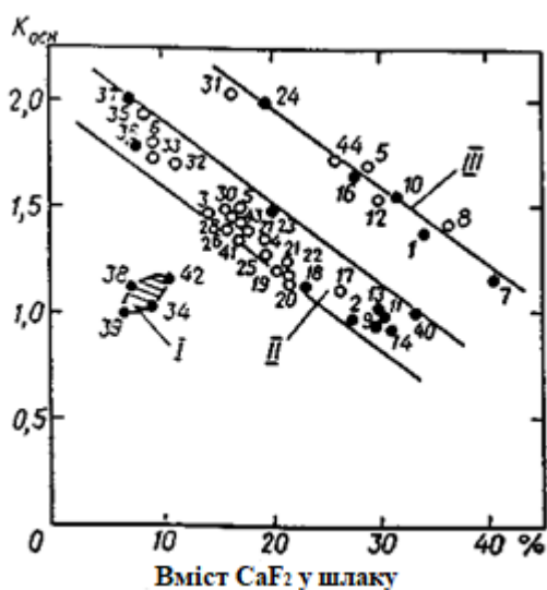
Рис. 2. Взаємозв'язок між кількістю \text{CaF}_2 у покритті та основи шлаку: • - закордонні електроди, о – вітчизняні електроди.
