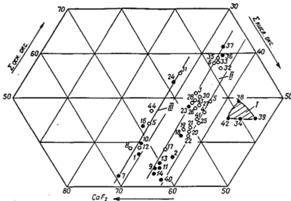
Рис. 1. Діаграма стану шлакової системи \text{CaO-CaF}_2\text{-SiO}_2\text{-TiO}_2 та області «оптимальної якості»: • - закордонні електроди, о – вітчизняні електроди.
