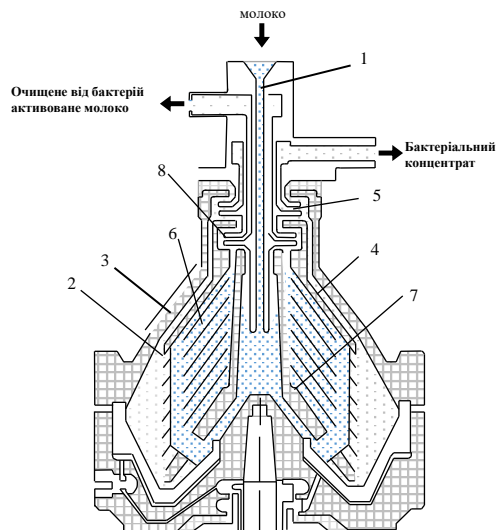
Рис.1 – Конструкція модернізованого сепаратора – очисника
