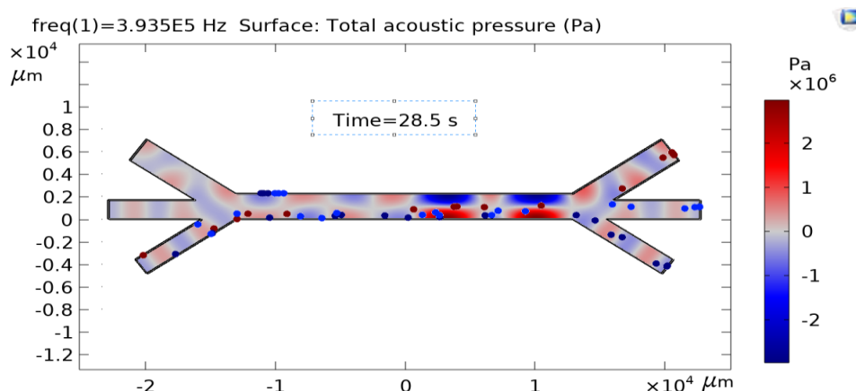
Рис.5. Розподіл часточок системі каналів під дією акустичної сили
