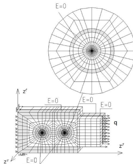
Рисунок 2 - Розрахункова схема НМСЕ
