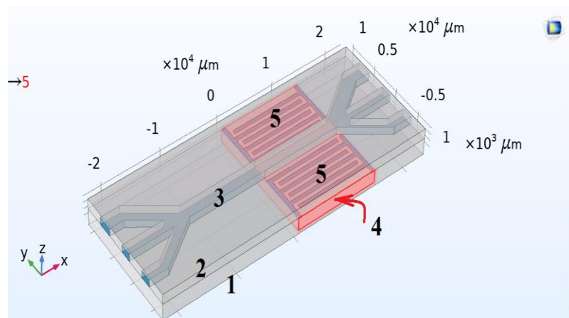
Рис. 1. Загальний вигляд мікросхеми для поділу трьох типів мікрочастинок: 1 – п'єзоелектричний матеріал \text{LiNbO}_3 ; 2 – зустрічно-штирьові перетворювачі; 3 – пластина з кремнію; 4 – мікрофлюїдний канал
