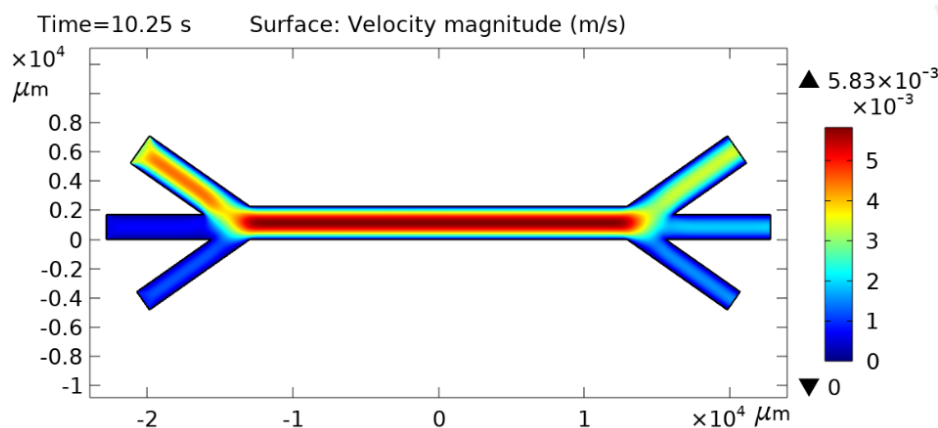
Рис. 2. Поле швидкостей для моделі з трьома вхідними каналами
