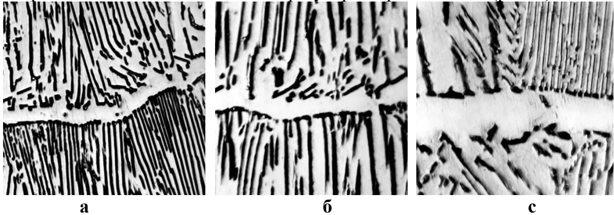
Рисунок 2. Структурні зміни на фронті росту аустенітно-карбідних колоній при зниженні температури в процесі науглецювання: а – \times 1000 , б – \times 1250 , в – \times 2000
