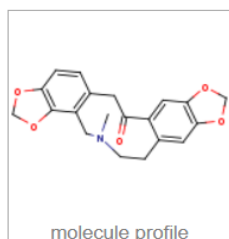
Рис.2. predictor – results активності протопіну на основі створеної моделі QSAR
