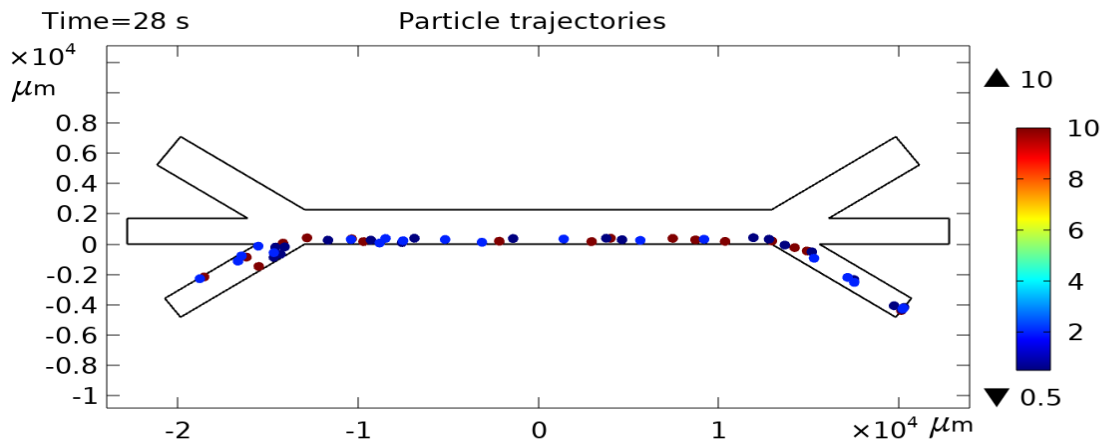
Рис. 3. Рух часточок без прикладеної акустичної сили
