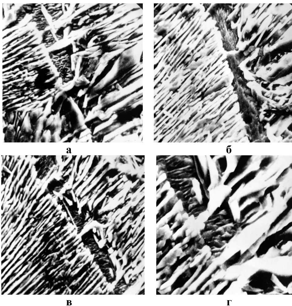
Рисунок 4. Сканувальна електронна мікроскопія дифузійного шару зразка сталі X20, науглецьованого в режимі термоцикування (1100...1000 °С). а, б, в – \times 1500 , г – \times 4000
