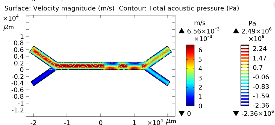
Рис. 4. Розподіл швидкостей з прикладеною акустичною силою
