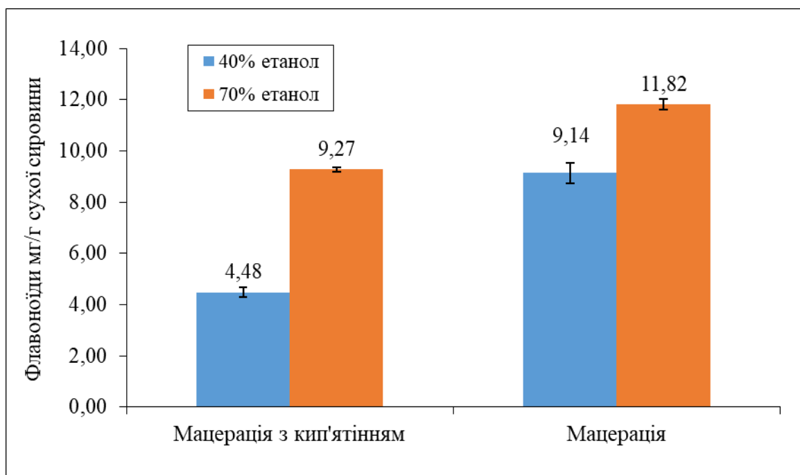
Рис. 1. Вміст флавоноїдів в екстрактах з листя Coriandrum sativum L. залежно від умов екстрагування
