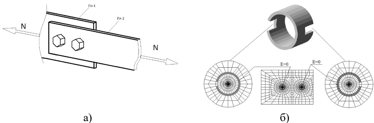
Рисунок 1- загальний вид (а), розрахункова схема МСЕ (б)
